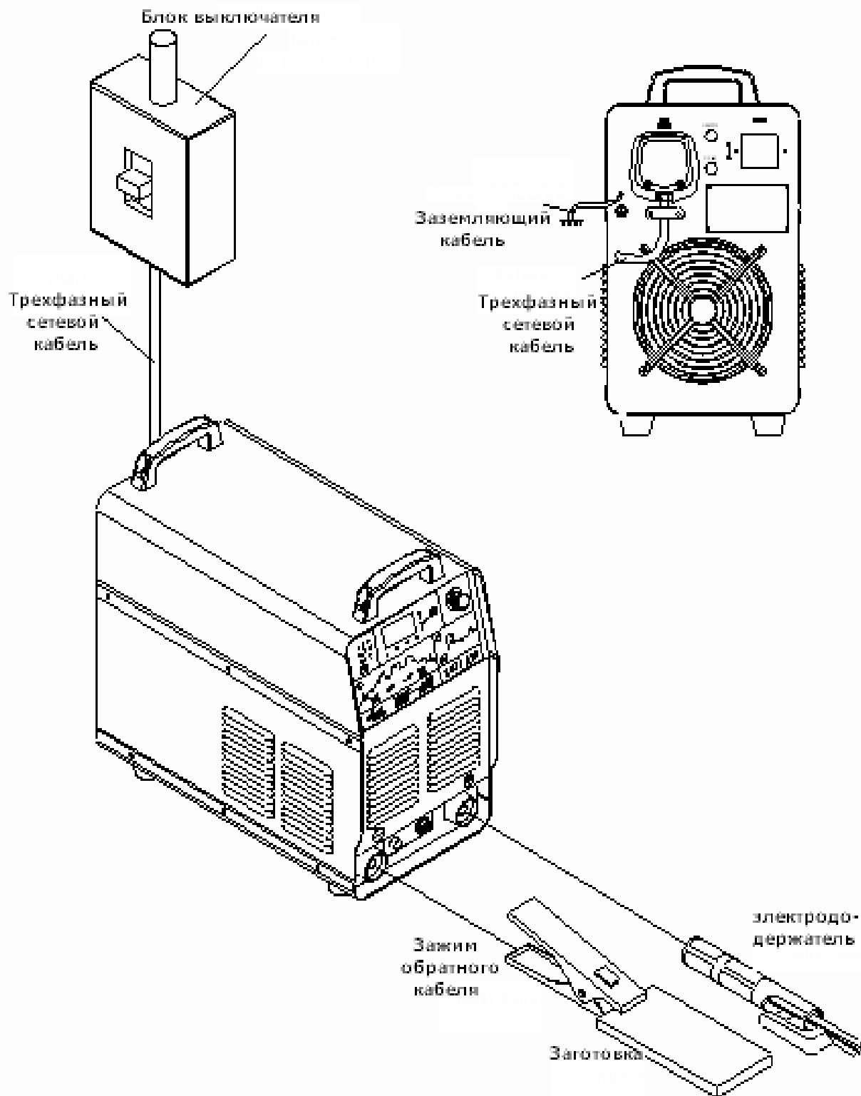
Рисунок 8.2 Сборка аппарата для режима сварки MMA – (справочно)
